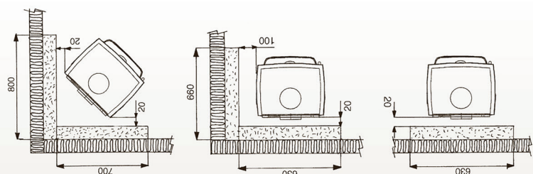
Utenpåliggende brannmur. Brannmurens høyde over ildstedet skal være min. 200 mm.
